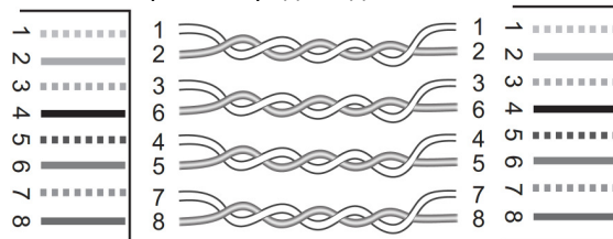
Схема подсоединения проводов при наличии расщепленных пар.
